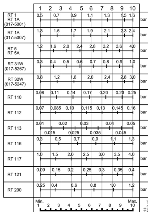
Рис. 8. Диаграмма выбора дифференциала
