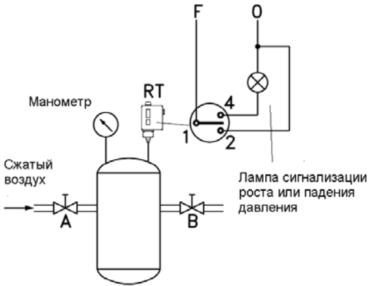
Рис. 9. пример использование реле давления с нейтральной зоной
