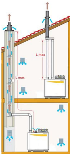
Примеры подключения
